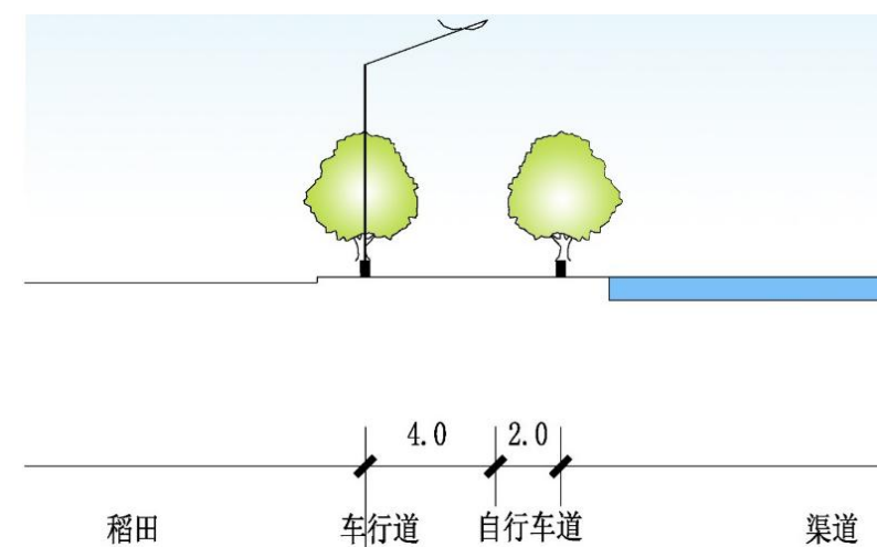
规划剖面
