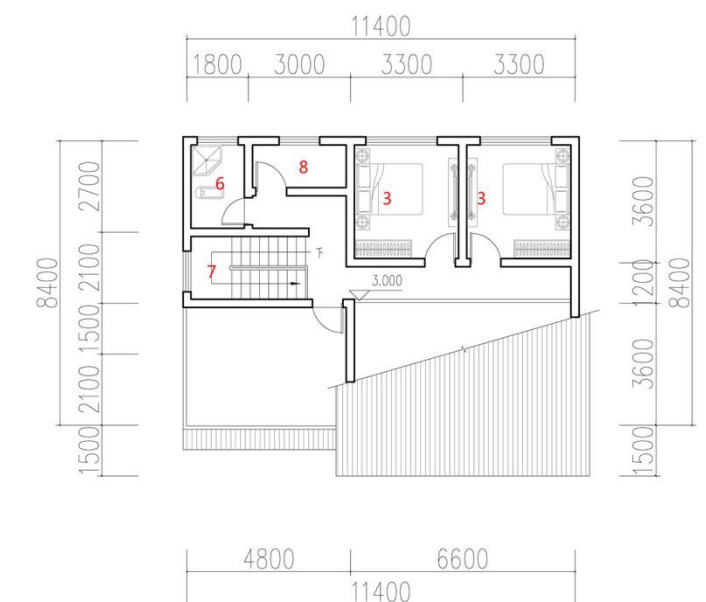
二层平面图
