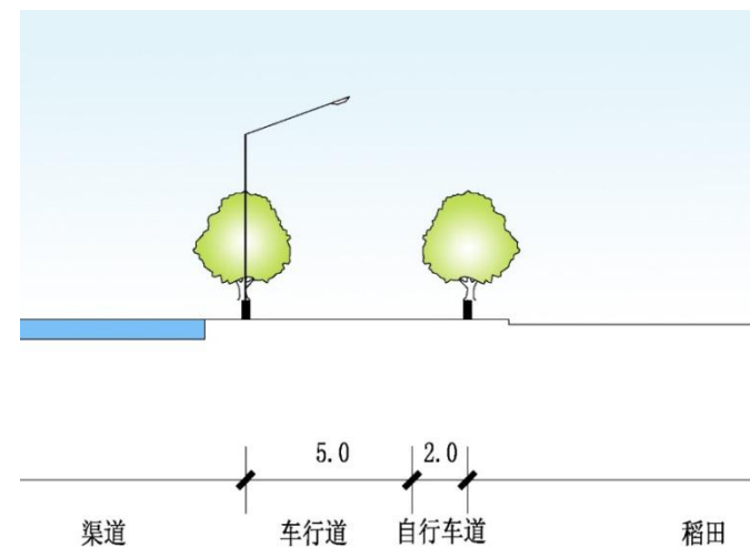
规划剖面
