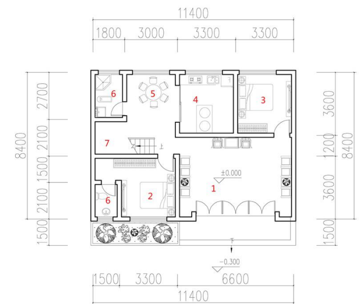
一层平面图
