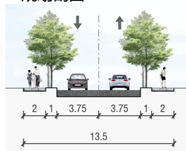
规划剖面
