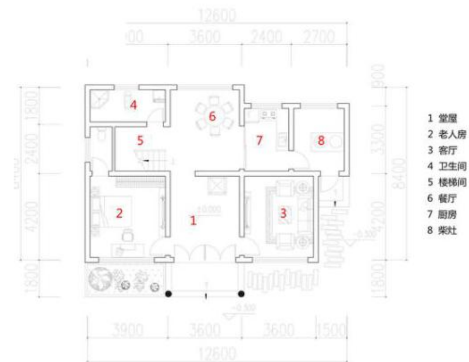
一层平面图
